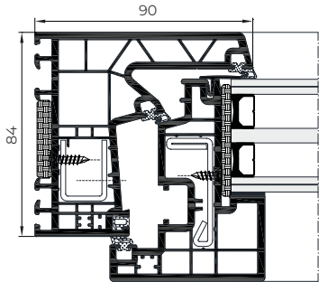
A 84 Hidden Sash Passivhausvhaus
